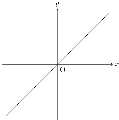
図1 一次関数のグラフ
