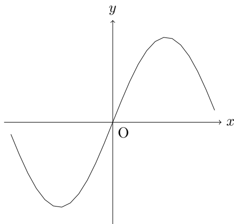
図3 三角関数(正弦波)のグラフ
