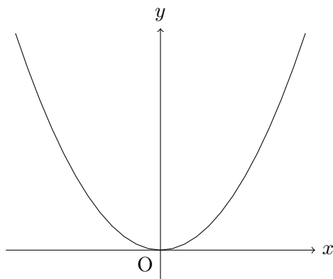
図2 二次関数のグラフ
